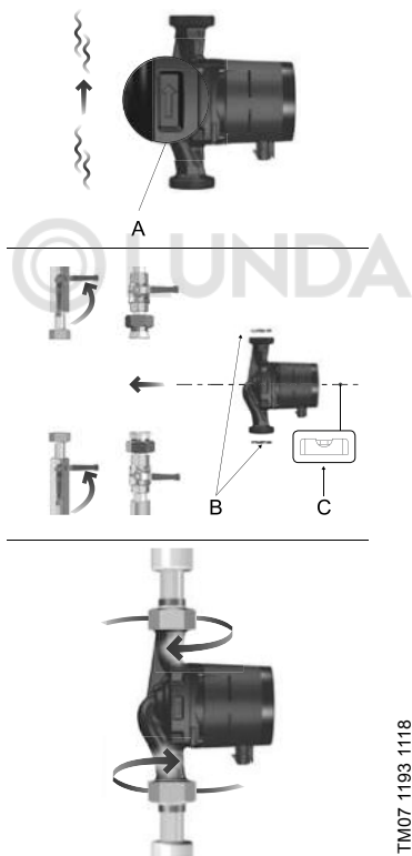
Рис. 3 Монтаж насоса ALPHA3
