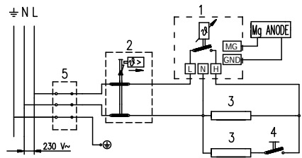
Электросхема
