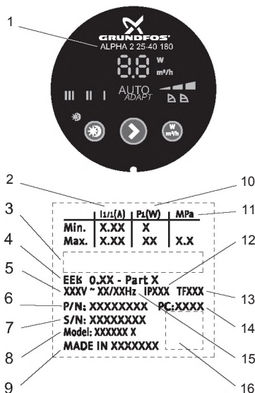
Рис. 2. Фирменная табличка
