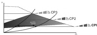
Рис. 23. Три кривые/настройки регулирования с постоянным давлением
