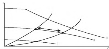
Рис. 25. Три настройки регулирования при фиксированной частоте вращения
