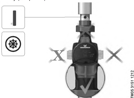
Рис. 8. Положение блока управления при монтаже насоса в системах кондиционирования и ХВС
