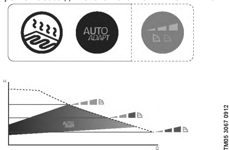
Рис. 22. Выбор настроек насоса в соответствии с типом системы . Заводская настройка: AUTO ADAPT .
