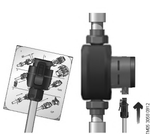
Рис. 12. Подключение к электросети
