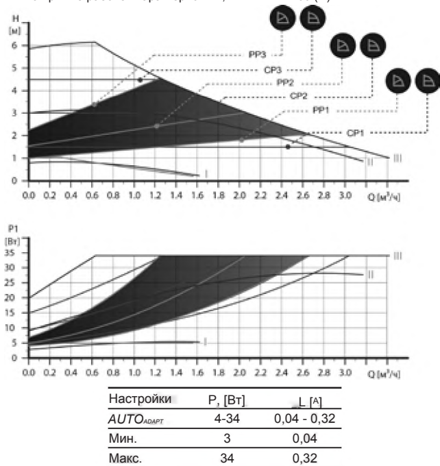
Рис. 34. ALPHA2 XX-60 (N)
