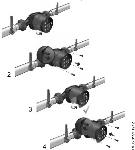
Рис. 9. Изменение расположения блока управления Блок управления можно поворачивать шагами по 90°.
