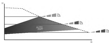
Рис. 20. Выбор настроек насоса в соответствии с типом системы
