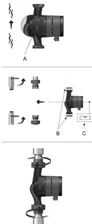
Рис. 5. Монтаж насоса ALPHA2
