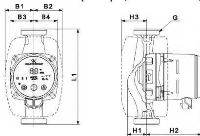
Рис. 29. ALPHA2 XX-40, XX-50, XX-60, XX-80
