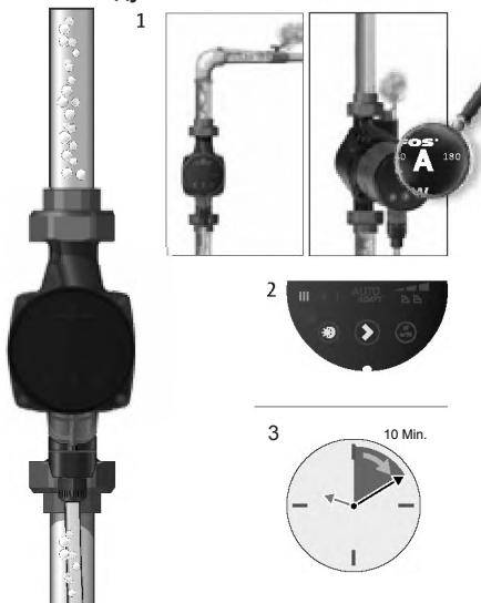
Рис. 15. Удаление воздуха из систем отопления
