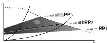
Рис. 19 Три кривые/настройки пропорционального регулирования
